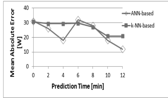
(d) MAE for W_{peak} = 350W (69 tests)
